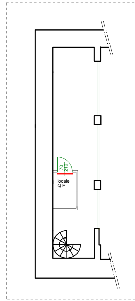
PIANTA SOPPALCO
