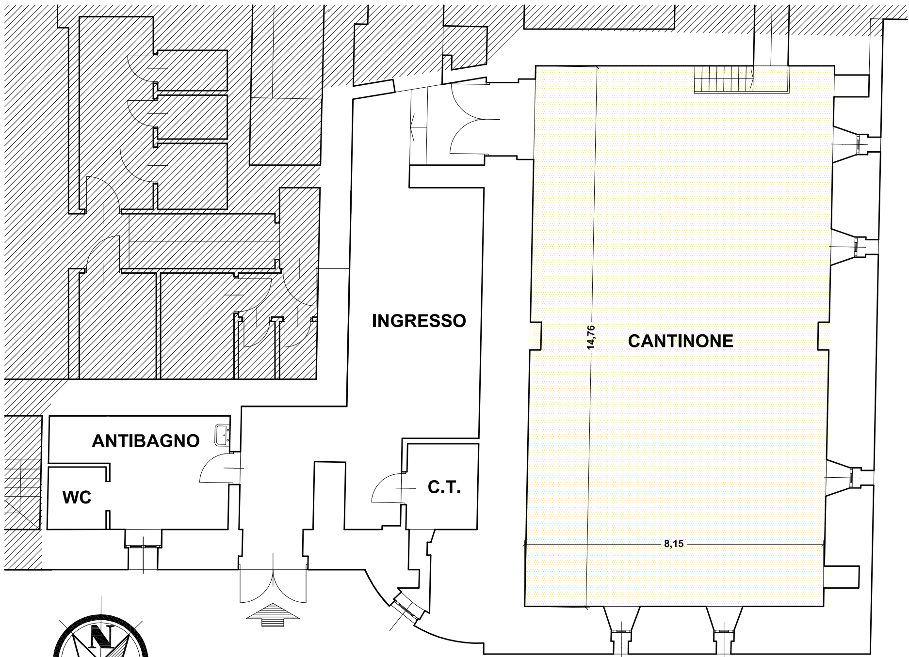
Castello Belgioioso Pianta Piano Interrato scala 1:100
