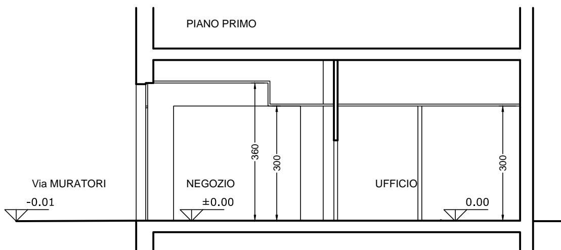
SEZIONE A-A
